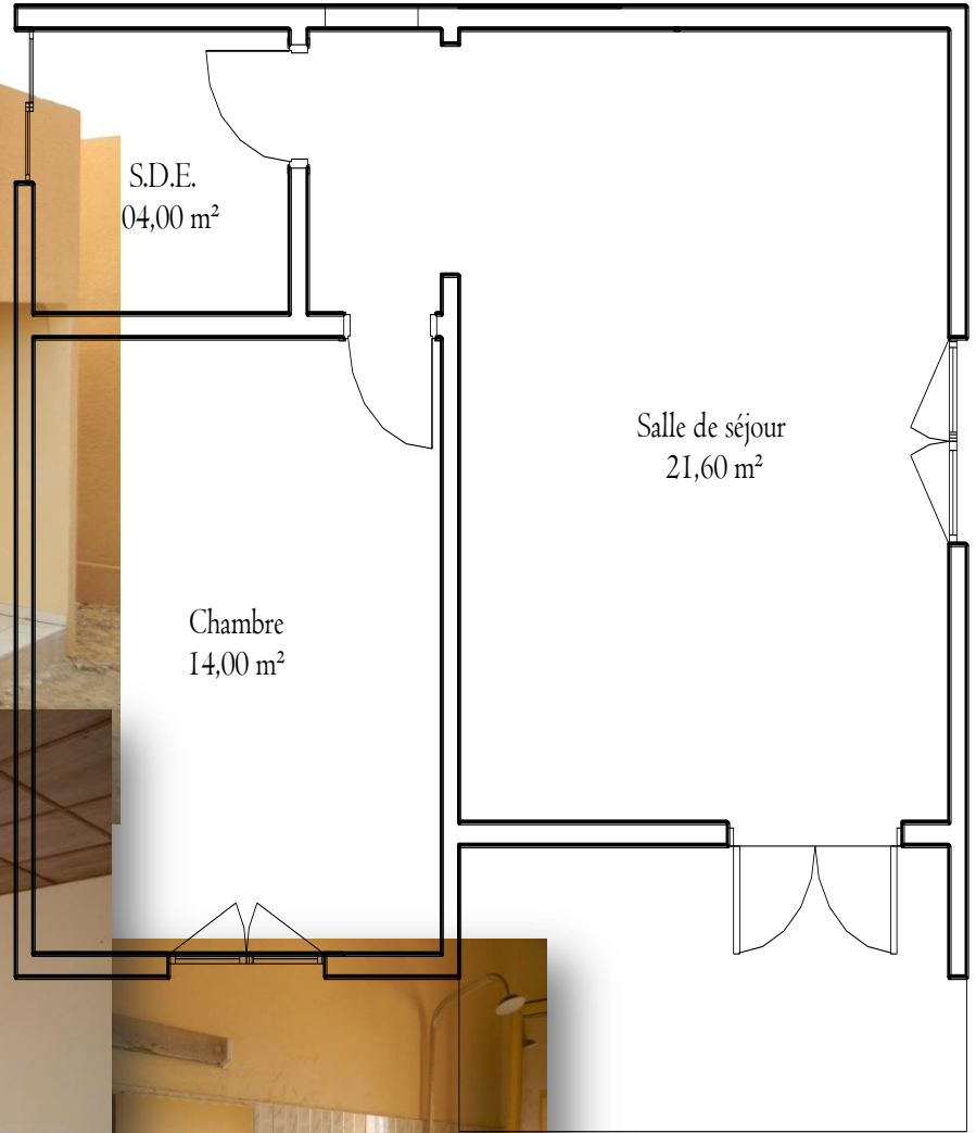
PLAN DE DISTRIBUTION Villa F2
